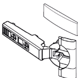
Blum scharnier 110° – volledig opliggend Blum Hinge 110° full overlay Blum charnière 110° recouvrement complète Blum scharnier 110° ganz aufrecht
